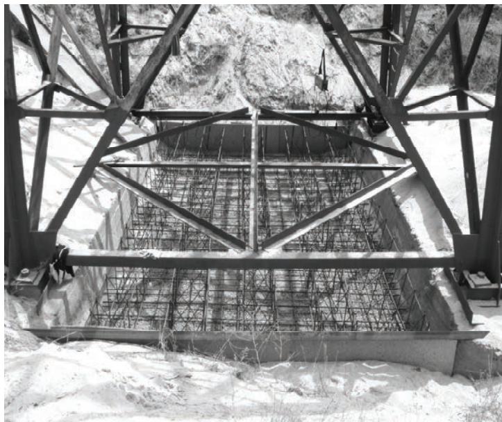
Рисунок 5. Усиление конструкций опор перехода ВЛ: а) увеличение сечения поясов; б), г) усиление фундаментов пригрузочными монолитными ростверками; в) локализация мест щелевой коррозии с обваркой узлов.
