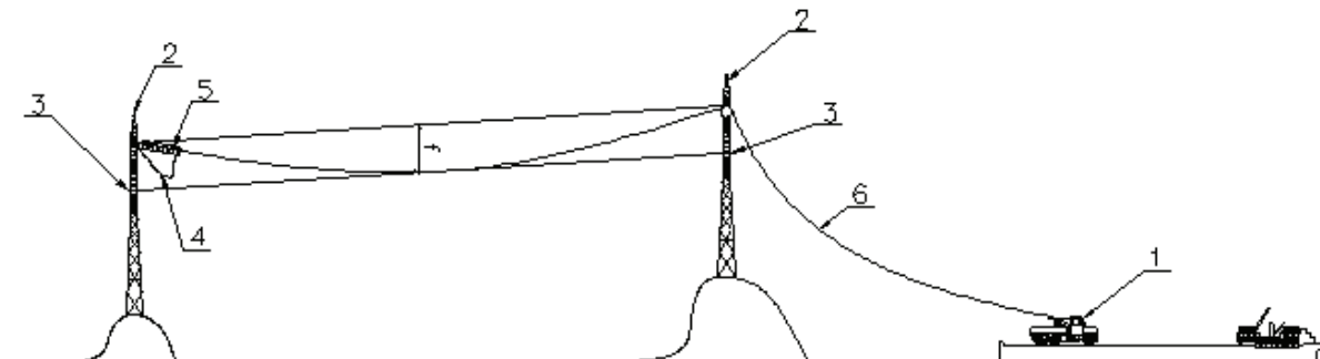
Рисунок 6. Натягивание и визирование проводов по стреле провеса: 1 – автомобиль с лебедкой на несамоходном судне; 2 – анкерная опора; 3 – визирная рейка; 4 – полупетля для обводного шлейфа; 5 – гирильнда изоляторов; 6 – натягиваемый провод (грозотрос).
