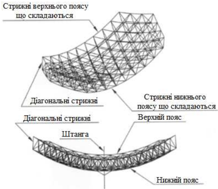
Рис.1. Просторова конструкція рефлектора антени
