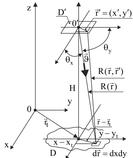
Рис. 1. Геометрия восстановления когерентных изображений поверхностей в зоне Фраунгофера
