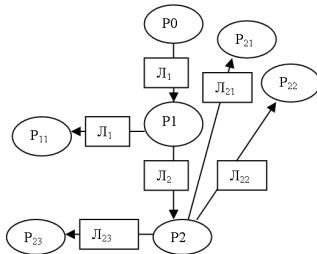
Рис. 2 – Пример радиальной сети
