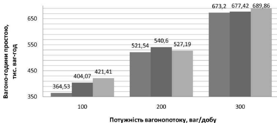
Рис. 1 – Сумарна тривалість знаходження вагонів на станції за варіантами технології обміну груп вагонів без зміни поїзного локомотива
