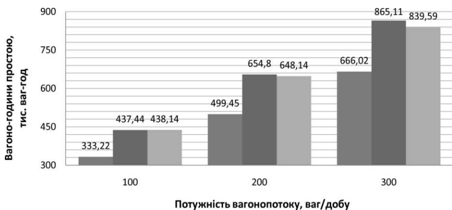
Рис. 2 – Сумарна тривалість знаходження вагонів на станції за варіантами технології обміну груп вагонів зі зміною поїзного локомотива
