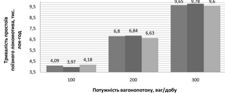
Рис. 5 – Сумарна тривалість простоїв поїзного локомотива на станції за варіантами технології обміну груп вагонів без зміни поїзного локомотива
