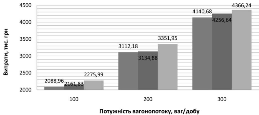
Рис.7 – Сумарні витрати на станції за варіантами технології обміну груп вагонів без зміни поїзного локомотива
