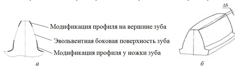
Рисунок 2 – Профильная и продольная модификация зубьев а – профильная модификация; б – продольная модификация
