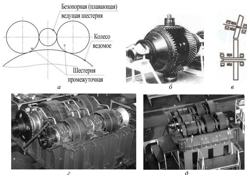
Рисунок 1 – Схемы и внешний вид некоторых запатентованных зубчатых передач а – замкнутое цилиндрическое зацепление с безопорной (плавающей) ведущей шевронной шестерней; б – замкнутая четырехшестеренная коническая передача с плавающей шестерней; в – эвольвентно-коническое (гиперболоидное) двухпоточное зацепление; з – двухпоточная косозубая передача; д – четырехпоточная косозубая передача
