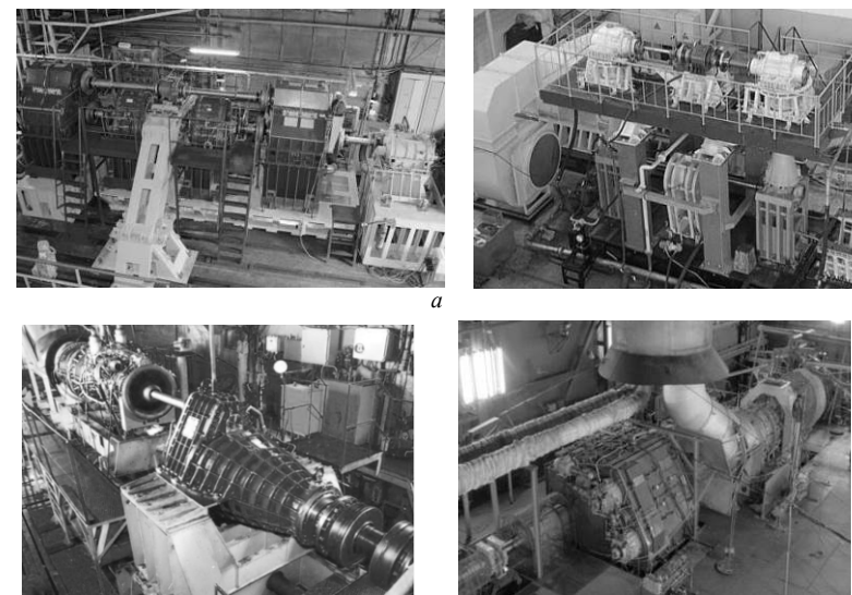
Рисунок 4 – Стенды для испытаний редукторов
