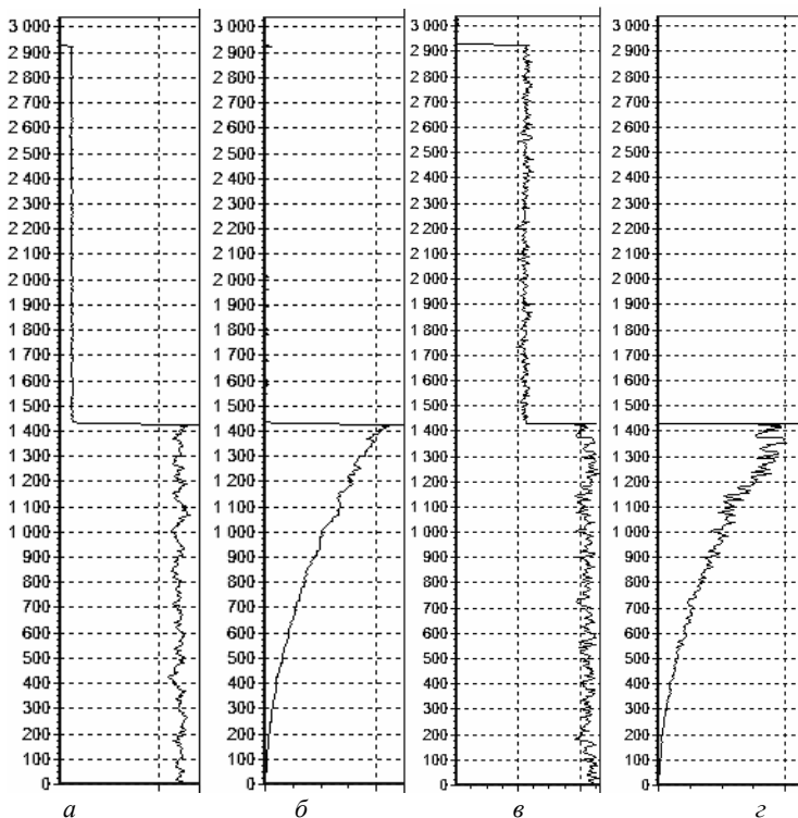
Рис. 5 – Мощность сигнала (а и в) и сечение рассеяния (б и г) для q=10 (а и б) и q=1 (в и г), усреднённые по 1464 радиолокационным развёрткам
