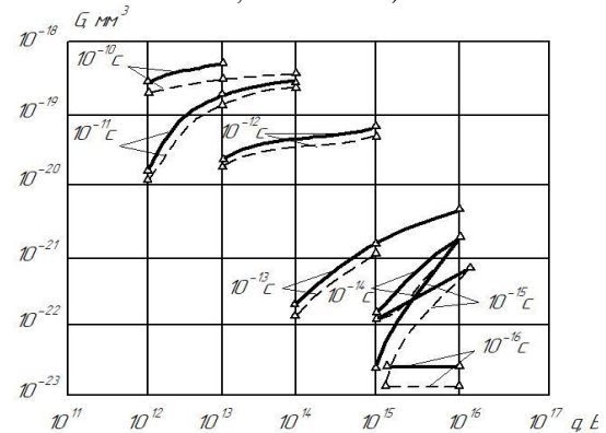
Рис. 3 – Зависимости объема, занятого наноструктурами, от плотности теплового потока q и времени для фемтосекундного лазера, действующего на Т12А (---) и Т23А (—) при R_p = 10^{-6} м
