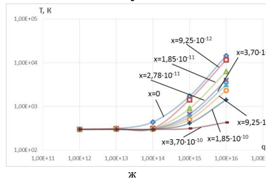
Рис. 2 – Продолжение (Зависимость максимальной температуры в зоне действия лазерного излучения на Т23А от плотности теплового потока на разных глубинах при времени действия: а - t=10^{-10} с; б - t=10^{-11} с; в - t=10^{-12} с; г - t=10^{-13} с; д - t=10^{-14} с; е - t=10^{-15} с; ж - t=10^{-16} с)
