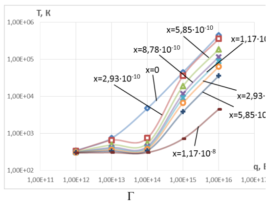
Рис. 2 – Зависимость максимальной температуры в зоне действия лазерного излучения на Т23А от плотности теплового потока на разных глубинах при времени действия: а - t=10^{-10} с; б - t=10^{-11} с; в - t=10^{-12} с; г - t=10^{-13} с; д - t=10^{-14} с; е - t=10^{-15} с; ж - t=10^{-16} с
