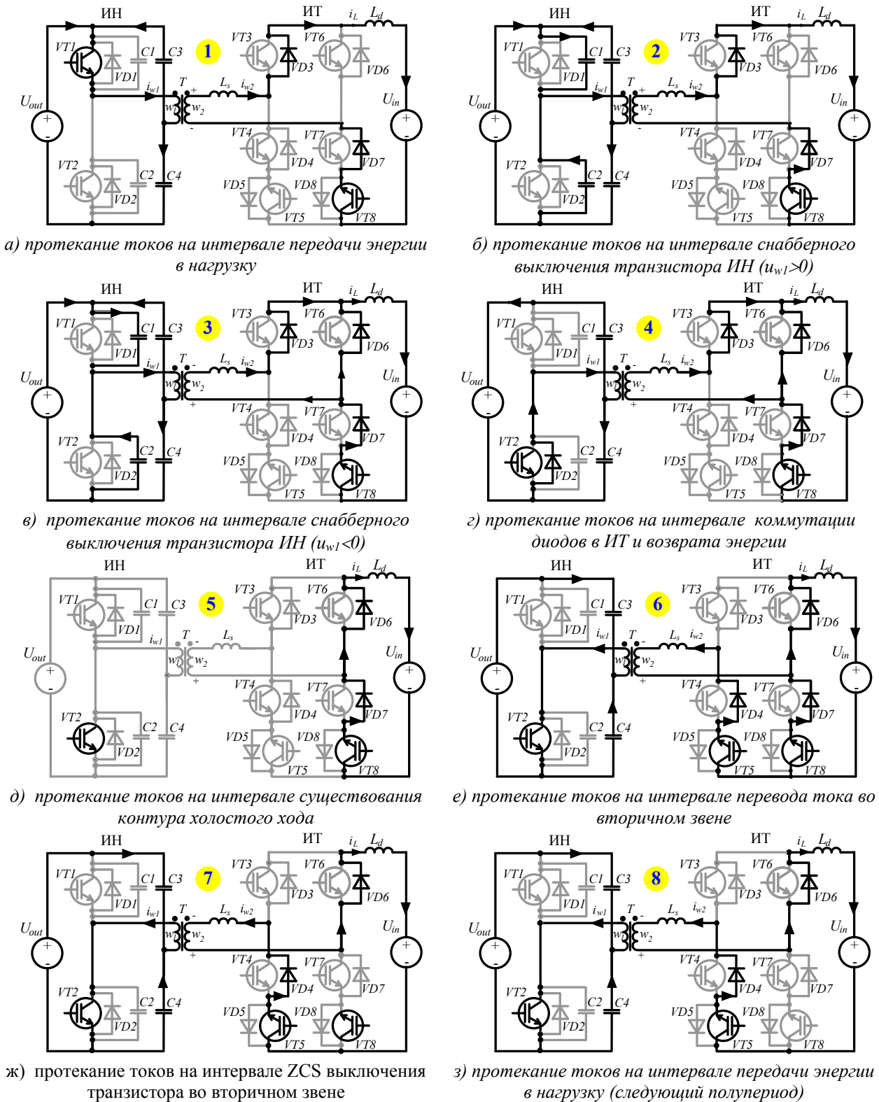
Рисунок 7. Пути протекания токов в ОАПРК на интервалах полупериода
