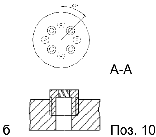
Рис. 4. Вібраційна змішувально - теплогенеруюча установка: а - загальний вигляд; б - розташування отворів (розріз А-А) та вигляд розетки змішувача-подрібнювача
