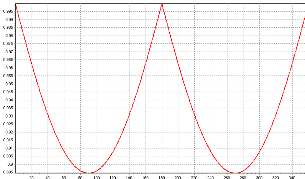
Рис. 4. Графік к.к.д. сферо-глобoidного сухарного синхронного карданного шарніра при \mu=0,3 , \alpha = 140^\circ , \gamma = 20^\circ
