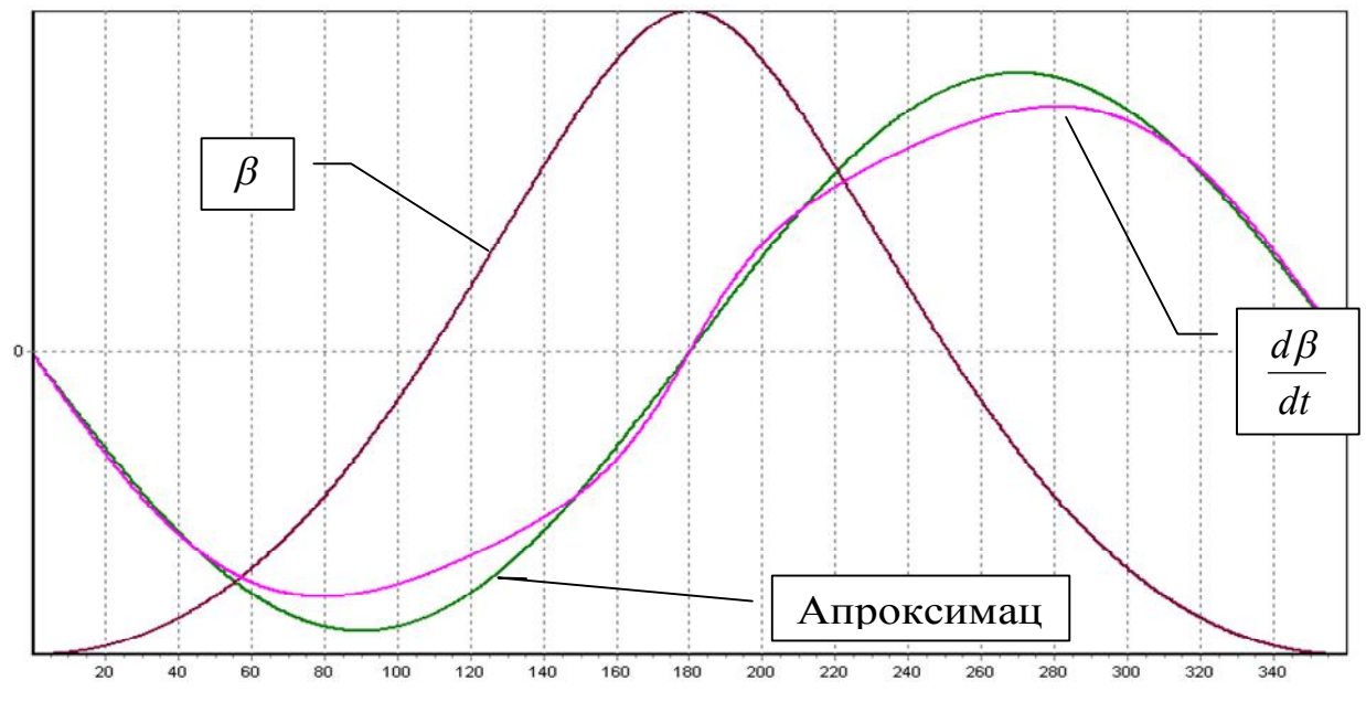
Рис. 3. Зміна кута \beta і кутової швидкості \frac{d\beta}{dt} від кута повороту ведучої ланки (при \alpha = 100^\circ , \gamma = 50^\circ , \omega = 1 ).
