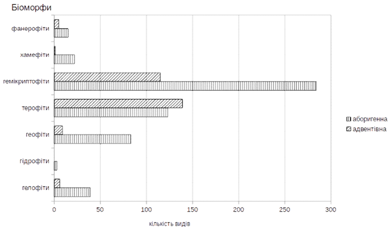
Рис. 1. Спектр біоморф ценофлори піонерної рослинності України.
