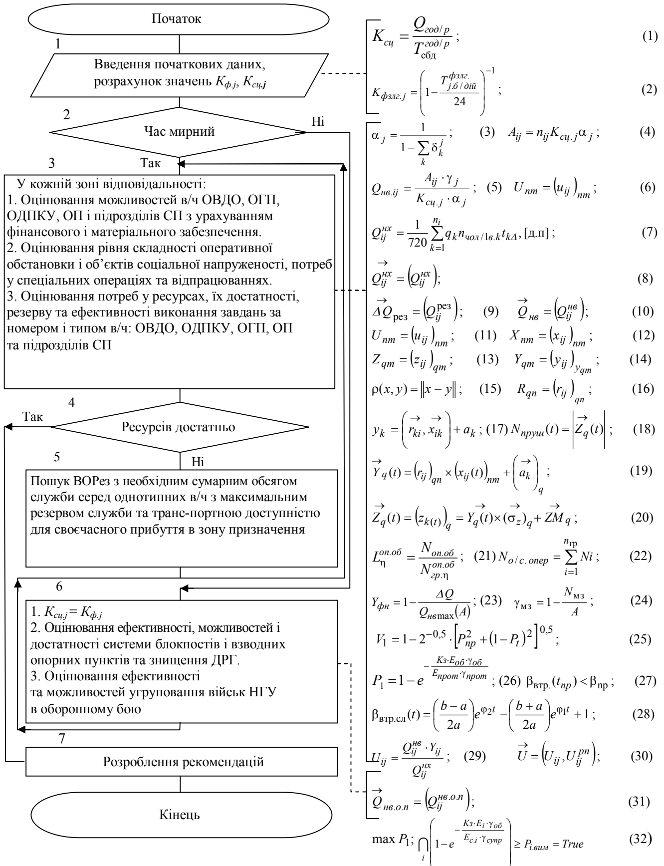
Схема алгоритму методу математичного моделювання й оцінювання ефективності та можливостей виконання службово-бойових завдань підрозділами, частинами і з'єднаннями Національної гвардії України
