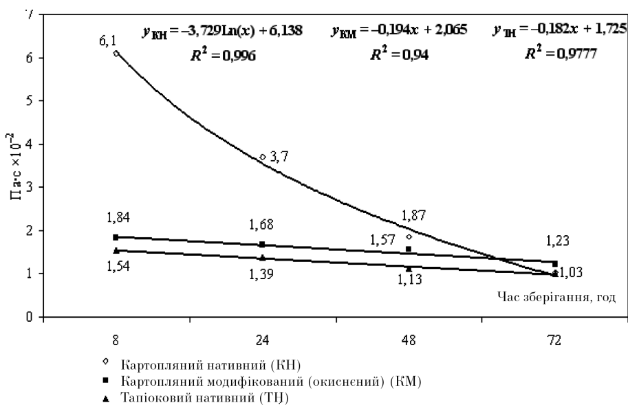
Рис. 4. Залежність в'язкості крохмальних клейстерів від часу зберігання
