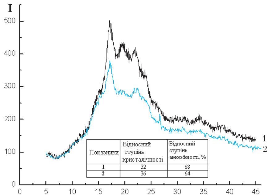
Рис. 3. Рентгенограми картопляного крохмалю: 1 – нативний; 2 – окиснений
