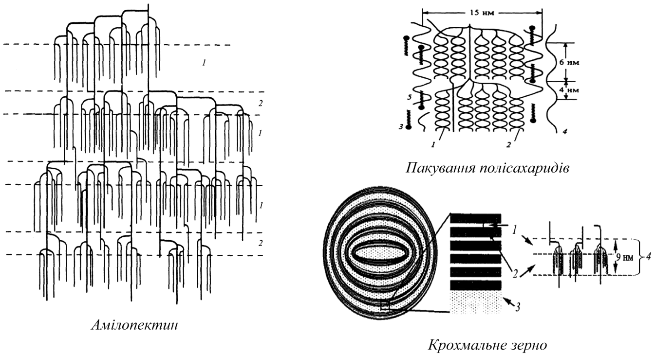
Рис. 2. Будова нативного крохмалю: амілопектин: 1 – кристалічні області, 2 – аморфні області; пакування полісахаридів: 1 – спіралі амілопектину, 2 – гібридні спіралі амілози та амілопектину, 3 – вільні ліпіди; 4 – вільна амілоза, 5 – V-структури амілози; крохмальне зерно: 1 – аморфна ламель, 2 – кристалічна ламель; 3 – аморфне ростове кільце; 4 – один кластер
