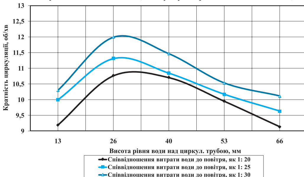
Рис. 2. Залежність кратності циркуляцій від витрат повітря і рівня води над циркуляційною трубою діаметром 118 мм
