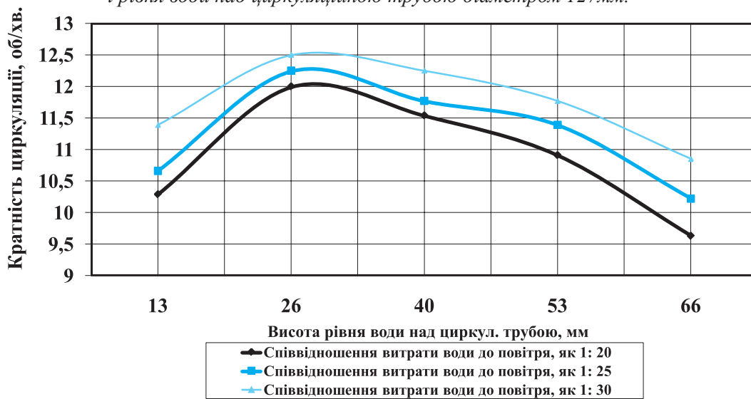
Рис. 4. Залежність кратності циркуляції від витрат повітря і рівня води над циркуляційною трубою діаметром 133 мм.
