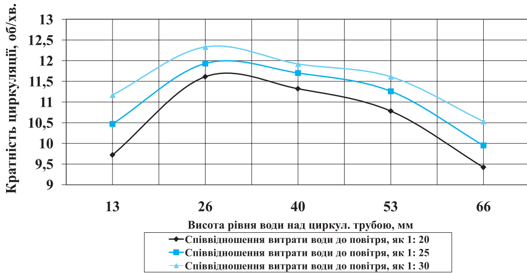
Рис. 3. Залежність кратності циркуляції від витрат повітря і рівня води над циркуляційною трубою діаметром 127 мм.
