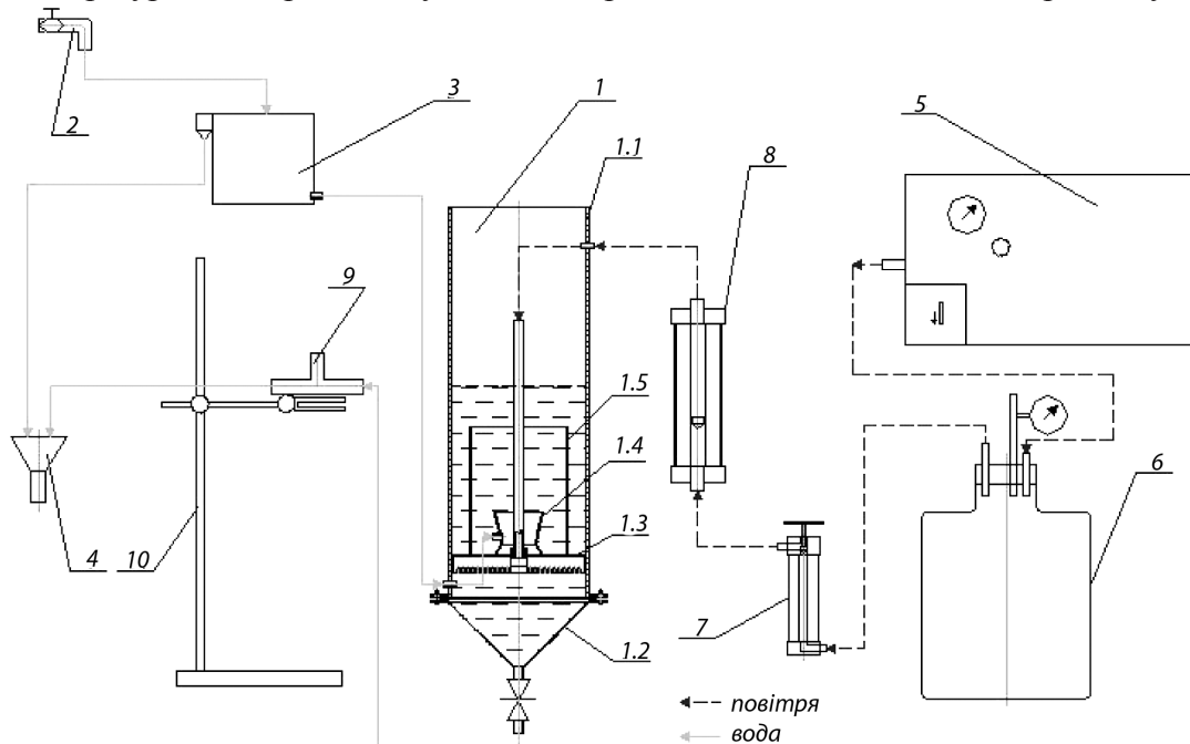
Рис. 1. Схема лабораторної установки: 1 - сатуратор (1.1- циліндричний корпус, 1.2 - конічне днище, 1.3 - барботер, 1.4 - карбонізатор, 1.5 - циркуляційна труба); 2 - кран; 3 - збірник-дозатор; 4 - лійка; 5 - компресор; 6 - накопичувач-ресивер; 7 - кран; 8 - ротаметр; 9 - пристрій; 10 - штатив.
