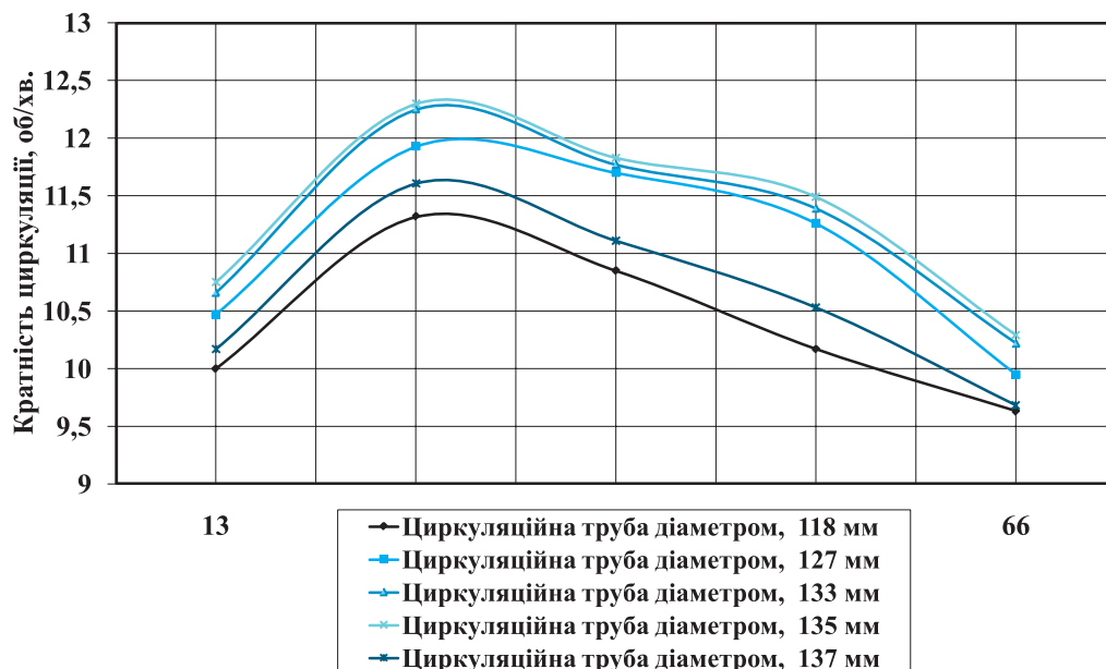
Рис. 5. Залежність кратності циркуляції від діаметра циркуляційної труби і рівня соку над нею при співвідношенні витрати газу до соку 25:1.
