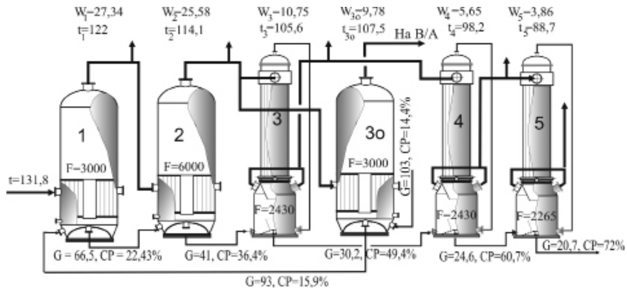
Рис. 3. Температурний режим на випарній установці з головними випарними апаратами Роберта та хвостовою частиною з плівковими випарними апаратами.
