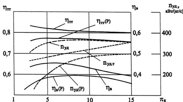
Рис.2. Зависимости КПД теплотехнического \eta_{ТТ} и внутреннего \eta_{в} соответственно удельных мощностей \eta_{уд,Т} и \eta_{уд,в} для ГТД с СТП и Р от изменения \pi_{к} при \sigma = 0,80 , \pi_{ДК} = 2,25 и T_3 = 1473 К.
