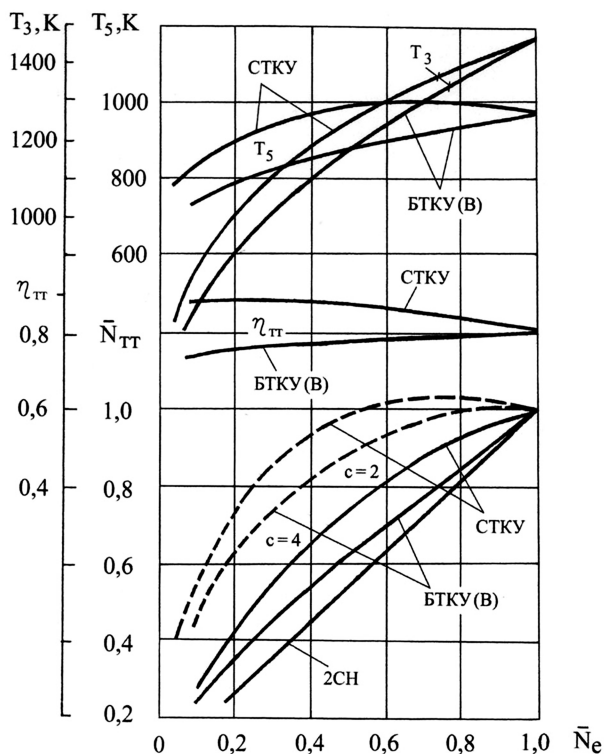
Рис.6. Теплотехнические характеристики ГТД с ТКУ и Р на частичных нагрузках при T_3 = 1473 К, \pi_c = 7 и \pi_{dk} = 2,25 (нагрузка винтовая): СТКУ – схема 1СН/Р со свободным ТКУ; БТКУ – схема 1СН/Р с заблокированным ТКУ.
