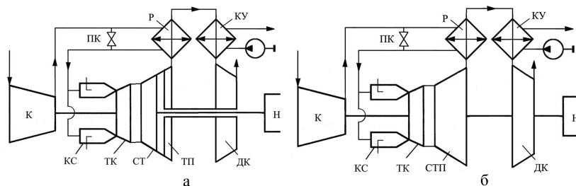
Рис.4. Когенерационный ГТД с ТКУ и регенерацией теплоты: а – схема со свободным ТКУ (схема 1СН/Р + СТКУ); б – схема с заблокированным ТКУ (схема 1СН/Р + БТКУ).
