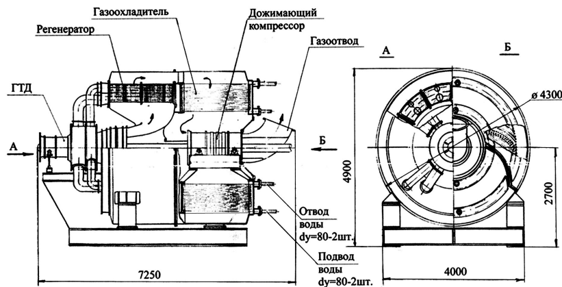
Рис.3. Когенерационный ГТД с ТКУ и регенерацией теплоты мощностью 10 МВт.
