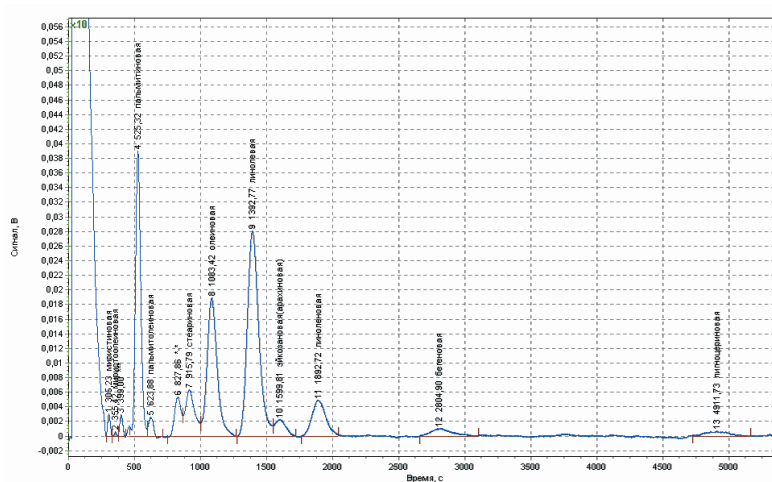
Рис. 3. Газова хроматограма жирнокислотного складу ліпофільної фракції кореневиць розогу вузьколистого
