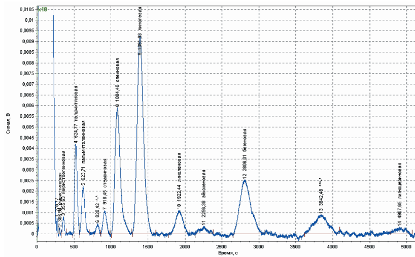
Рис. 2. Газова хроматограма жирнокислотного складу ліпофільної фракції плодів розогу вузьколистого
