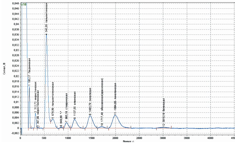
Рис. 1. Газова хроматограма жирнокислотного складу ліпофільної фракції листа розогу вузьколистого
