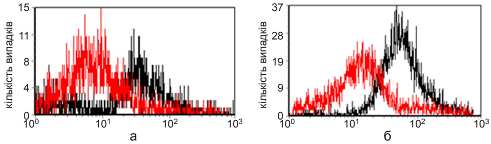
Рис. 2. Інтенсивність флуоресценції бузини чорної-SNA (а) і маакії амурської-MAА II (б) на лімфоцитах гематологічно здорового донора (світла лінія) і хворого на еритремію (темна лінія), протокова цитометрія на апараті («Beckman Coulter EPICS»)
