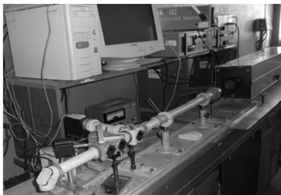
Рис. 4. Программируемый амплитудный модулятор, установленный в квазиоптическом тракте
