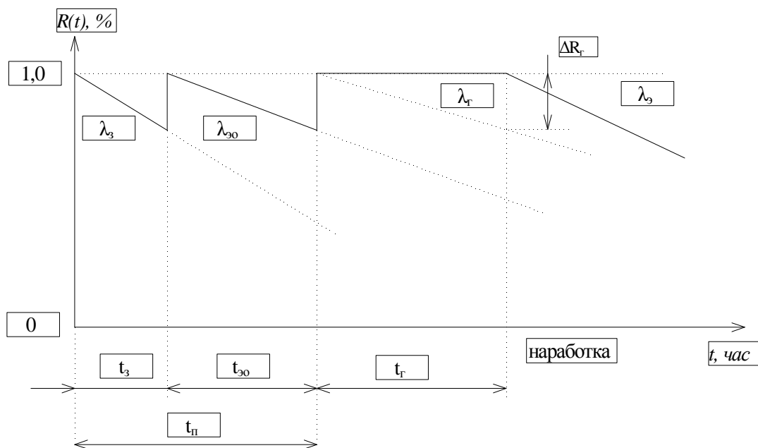
Рис. 1. Графическая модель безотказности нового и отремонтированного изделия в период производственных испытаний: t_{30} – эксплуатационные испытания; t_n – период передаточных испытаний (приработка); t_r – период гарантийной эксплуатации (гарантийная надежность эксплуатации).
