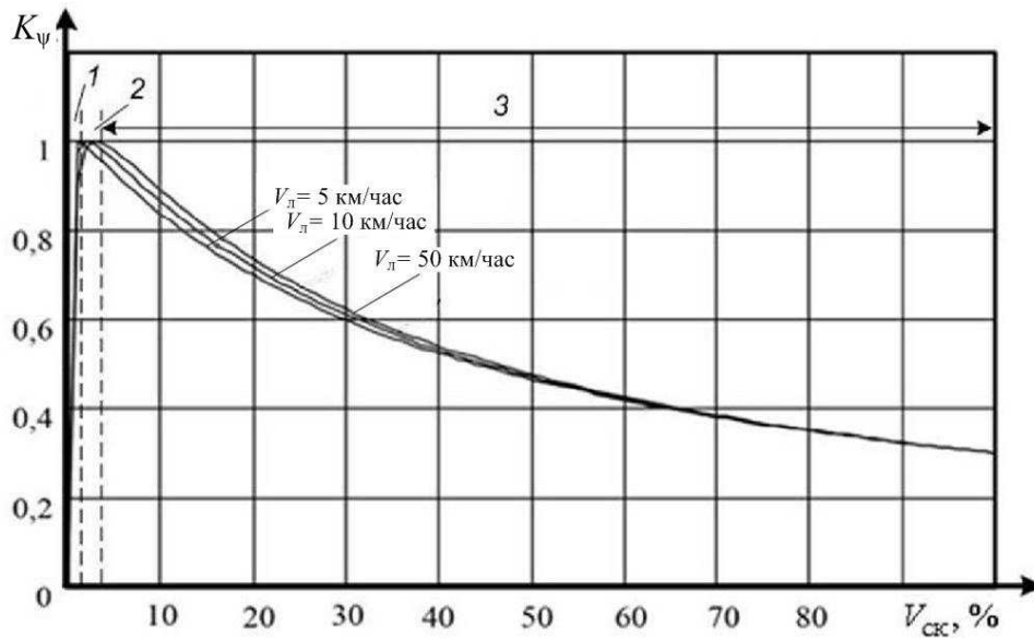
Рис. 7. Характеристика сцепления
