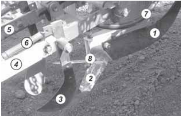
Рис. 1. Усовершенствованная посевная секция сеялки СУПН-6А, оборудованная стрельчатым УС для ЛВВГ: 1 – полоз сошника; 2 – УС; 3 – загортак; 4 – удлинитель тяги; 5 – тяга; 6 – пружина привода загортача; 7 – канал для подвода рабочей жидкости, 8 – распылитель.
