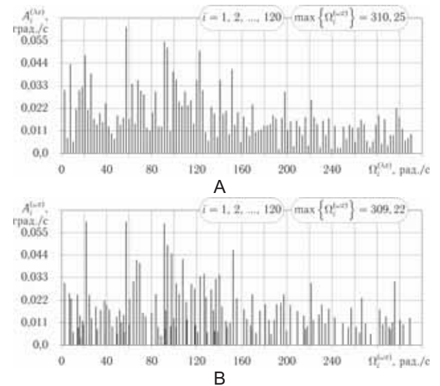
Рис. 8. Амплитудно-частотный спектр ( \Omega_i^{(\omega z)} — частота, рад./с; A_i^{(\omega z)} — амплитуда, град.): А) функции \omega_z(t) (град./с, кривая 2, рис. 6.) интерполяции точек данных измерения угловой скорости посевной секции в случае применения ППФ, когда задействованы все n = 120 гармоник; В) функции \omega_z(t) (град./с) аппроксимации тех же данных путем применения ПП, когда максимальное значение частоты \max\{\Omega_i^{(\omega z)}\} и число гармоник соответствуют предыдущему варианту
