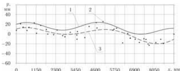
Рис. 10. Результаты восстановления линии рядка: 1 и 3 — фактическая и восстановленная линия рядка; 2 — точки семян давших всходы
