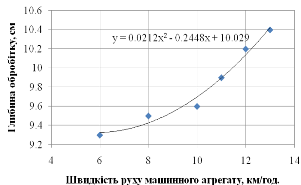
Рис. 7. Зміна глибини дискування при зміні швидкості руху машинного агрегату у складі New Holland + Quivogre APXTL 36
