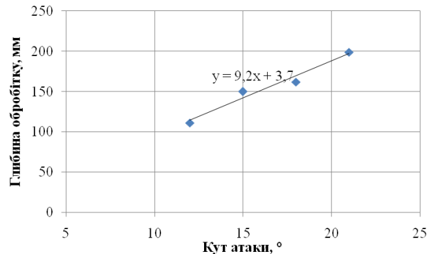
Рис. 12. Зміна глибини дискування при зміні кута атаки машинного агрегату у складі МТЗ-892 + УДА-2,4
