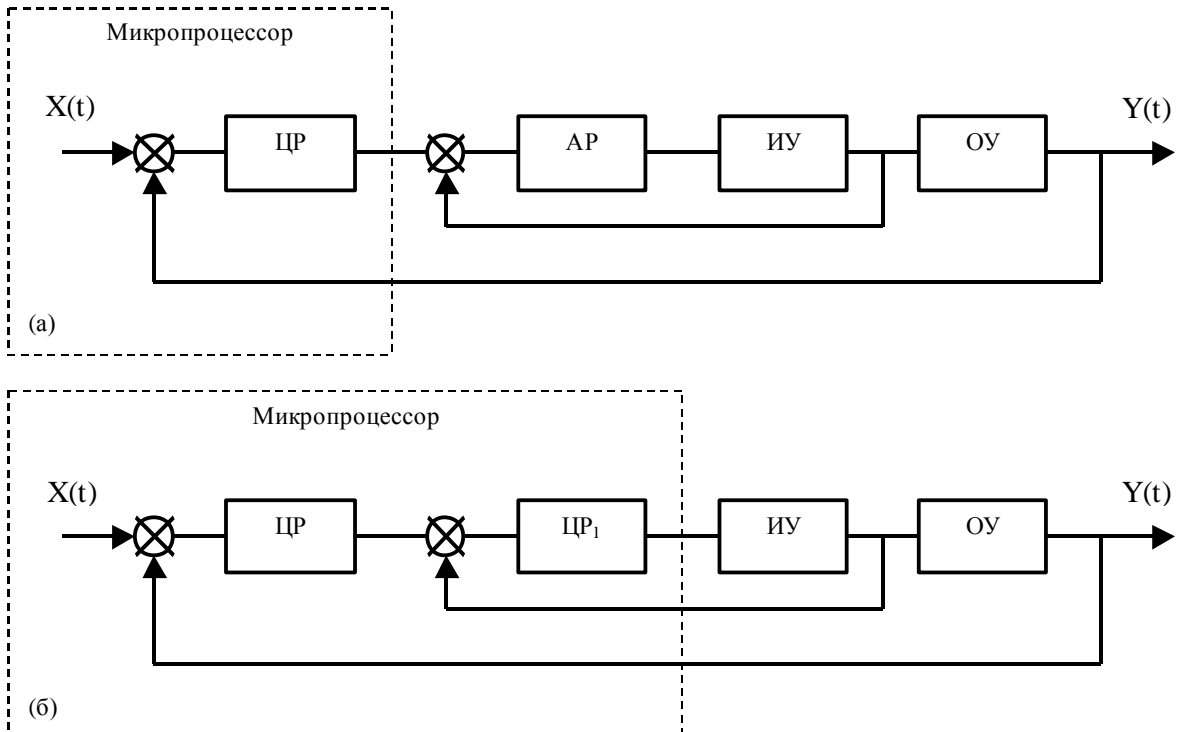
Рис. 6. Структурная схема САУ компенсирующая нелинейности ИУ: а) ССУ; б) СУсСИУ. АР – аналоговый регулятор
