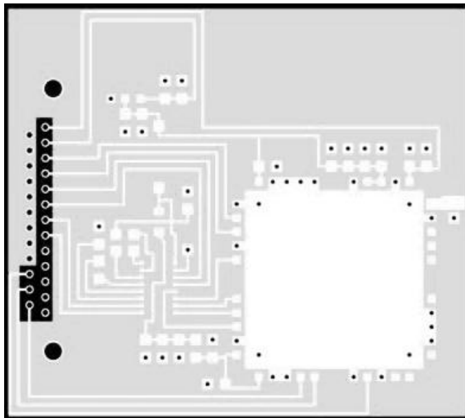
Рис. 3. Друкована плата бортової складової СОНІМ
