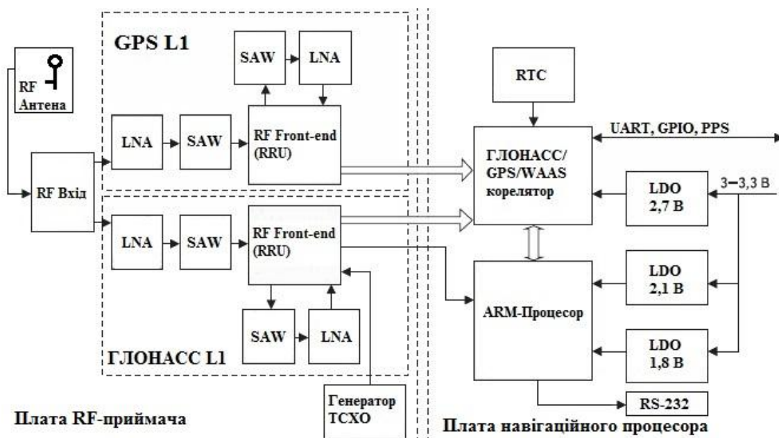
Рис. 1. Функціональна схема бортової частини СОНІМ RF Front-end (RRU) – надвеликі інтегральні схеми радіоприймального пристрою.
