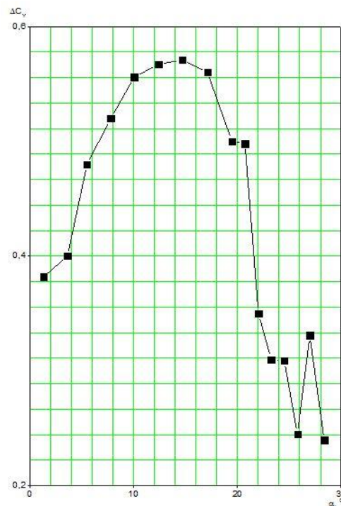
Рис. 2. Экспериментальная модель крыла [4]. Влияние деформаций крыла на коэффициент подъемной силы по углу атаки. Зависимости \Delta C_y=f(\alpha, \text{ХЖЧ}) . Re = 222603 ; M = 0,073
