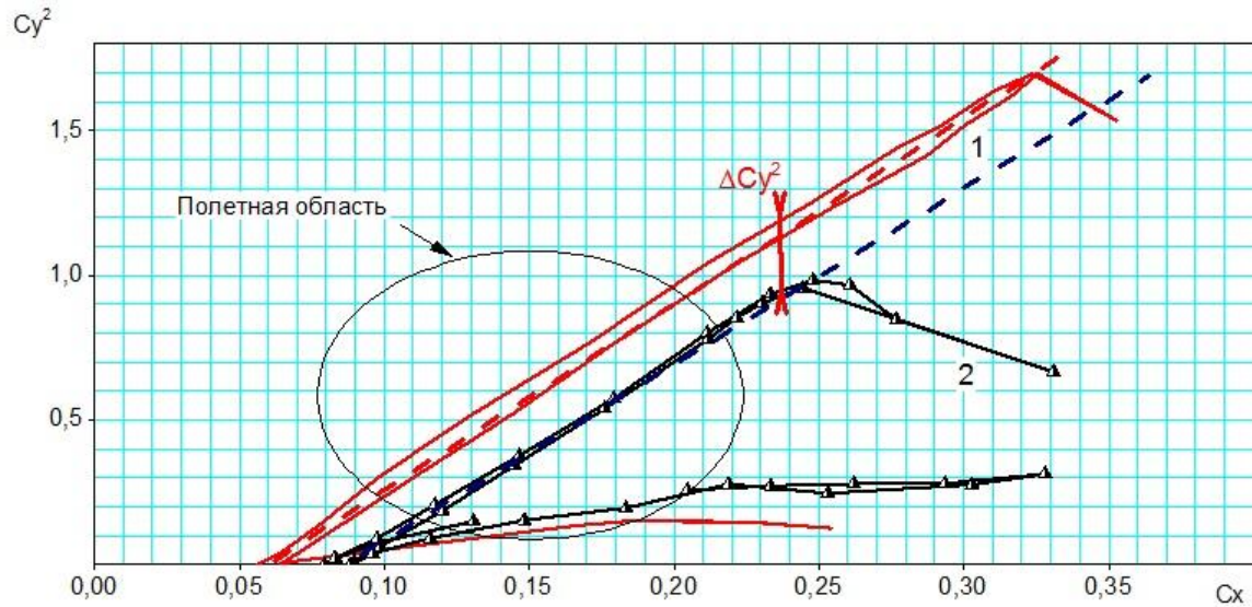
Рис. 3. Экспериментальная модель крыла [4].
