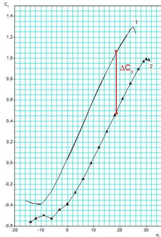
Рис. 1. Экспериментальная модель крыла [4]. Зависимости C_y=f(\alpha, \text{ХЖЧ}) . Re = 222603 ; M = 0,073 ; 1 – жесткое крыло; 2 – жесткая часть 30% хорды
