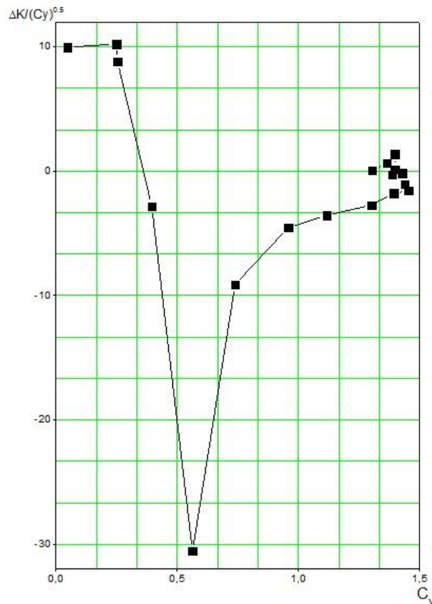
Рис. 8. Экспериментальная модель крыла [4]. Влияние деформаций крыла на критерий максимальной дальности для различных значений коэф-та подъемной силы. Зависимости \Delta K/(C_y)^{0.5} = f(C_y, \text{ХЖЧ}) . Re = 222603 ; M = 0,073
