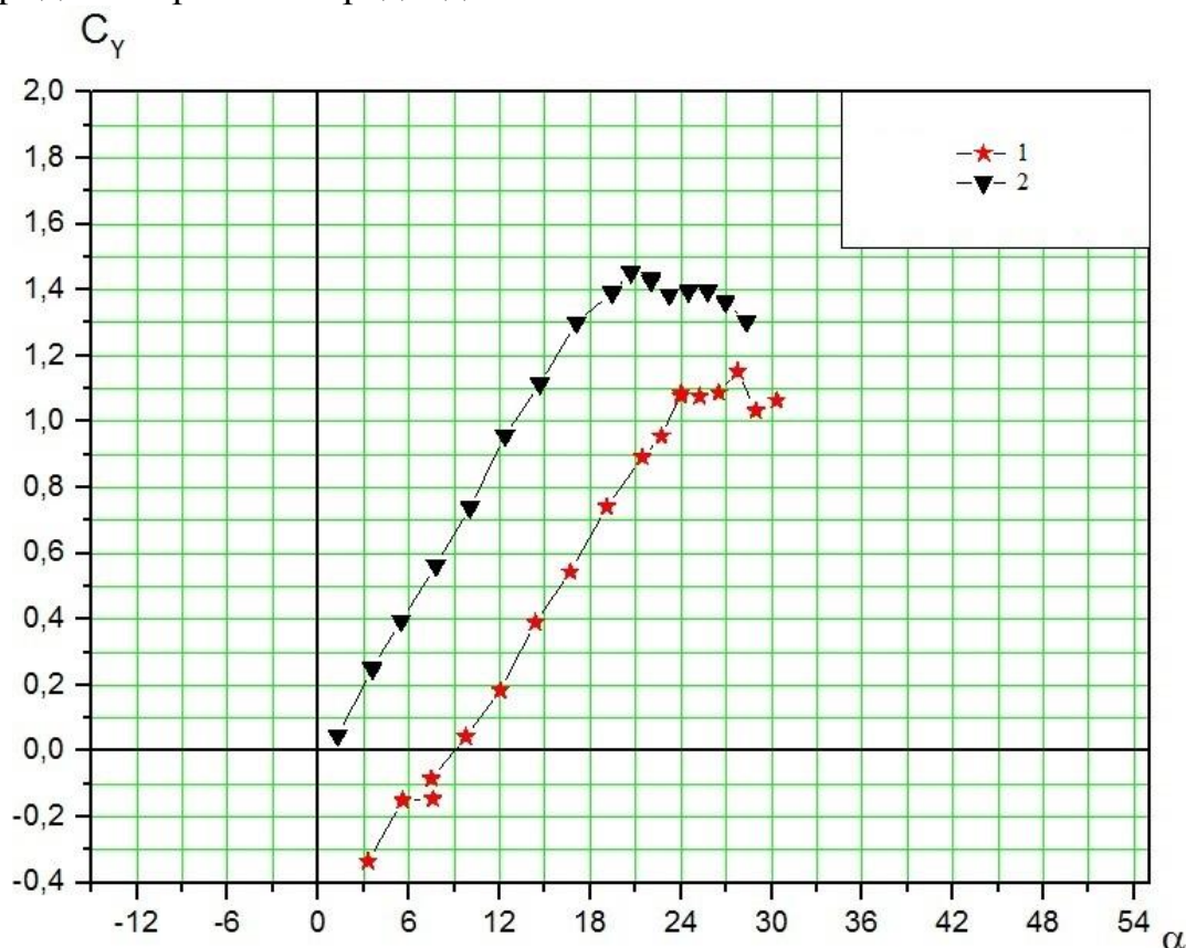
Рис 9. Модель А-20. Зависимость C_y = f(\alpha) .
