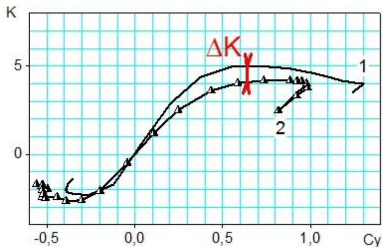
Рис. 5. Экспериментальная модель крыла [4]. Зависимости K=f(C_y, \text{ХЖЧ}) . Re = 222603 ; M = 0,073 ; 1 – жесткое крыло; 2 – жесткая часть 30% хорды
