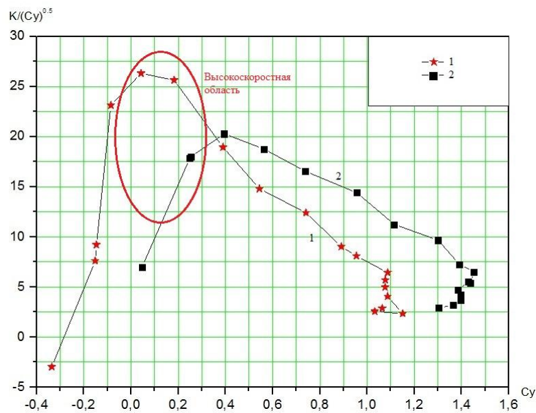
Рис. 11. Модель А-20 Зависимость K = f(C_y) .
