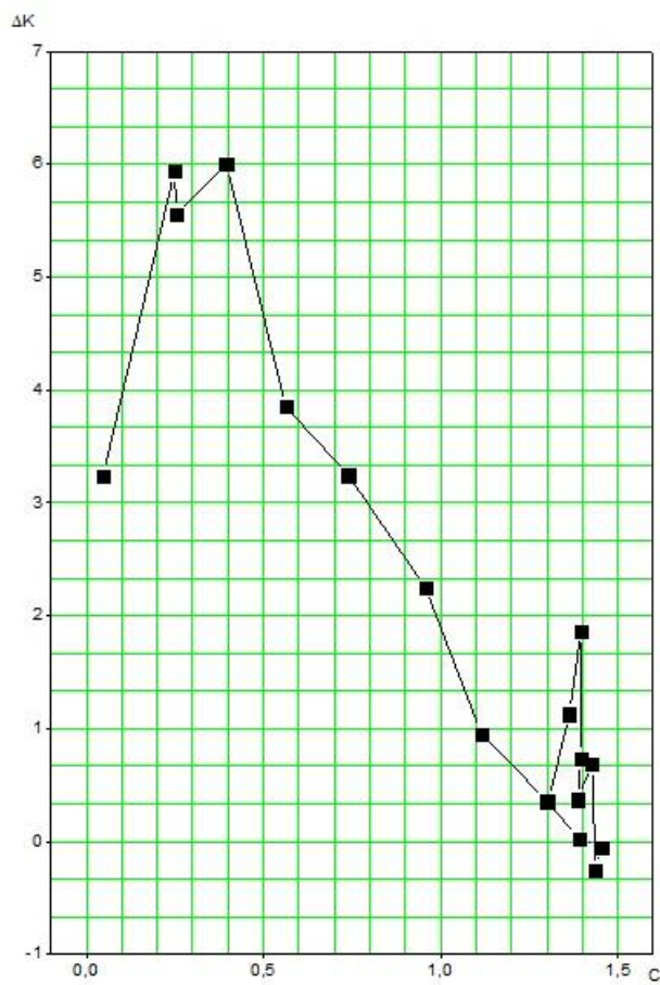
Рис. 6. Экспериментальная модель крыла [4]. Влияние деформаций крыла на аэродинамическое качество K для различных C_y . Зависимости \Delta K=f(C_y, \text{ХЖЧ}) . Re = 222603 ; M = 0,073
