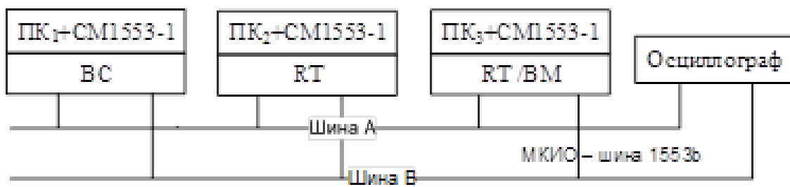
Рис. 4. Схема моделирующей системы авионики
