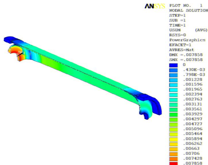
Рис. 5. Суммарные перемещения системы, м
