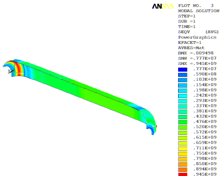
Рис. 9. Эквивалентные напряжения, Па
