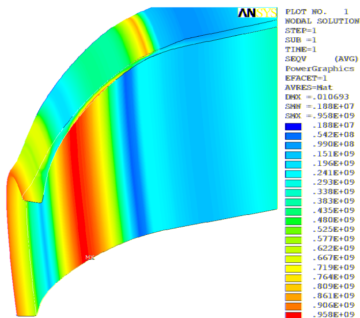
Рис. 12. Эквивалентные напряжения, Па
