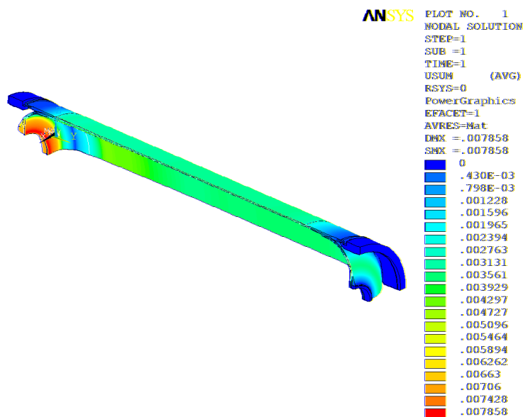
Рис. 3. Суммарные перемещения системы, м
