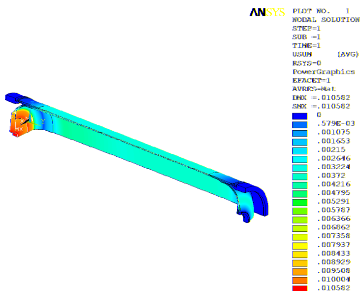
Рис. 8. Суммарные перемещения системы, м
