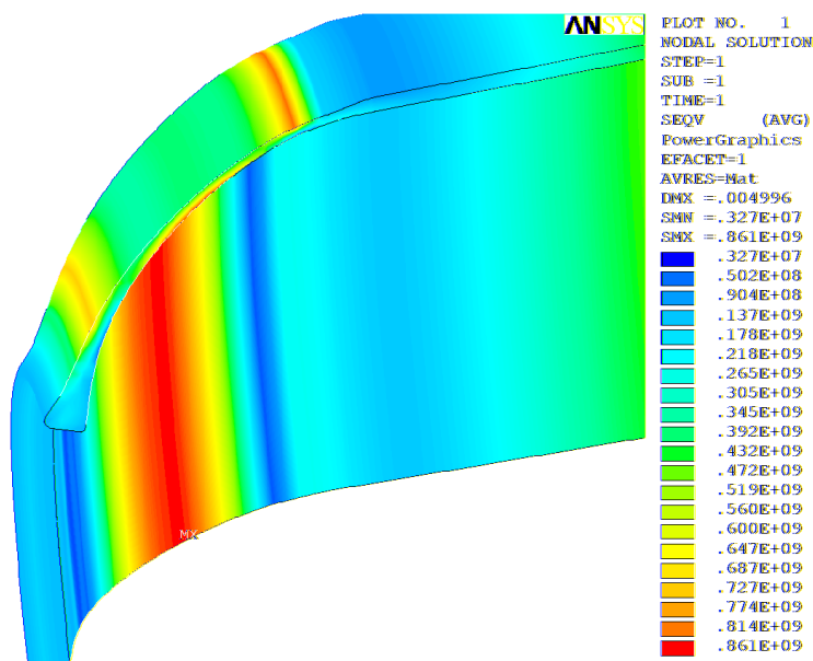
Рис. 14. Эквивалентные напряжения, Па
