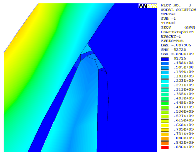
Рис. 7. Эквивалентные напряжения, Па
