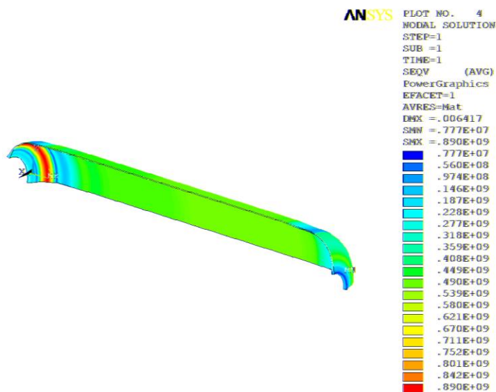
Рис. 6. Эквивалентные напряжения, Па
