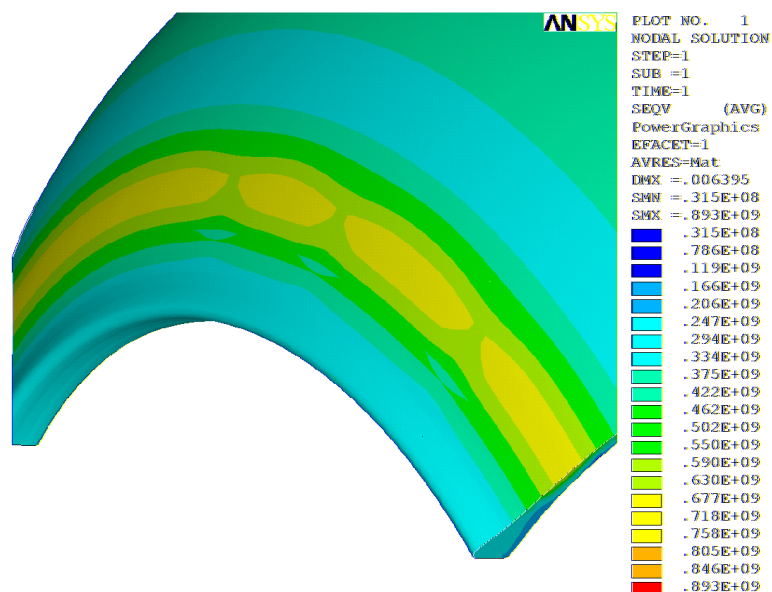
Рис. 11. Эквивалентные напряжения, Па
