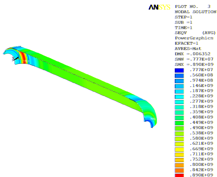
Рис. 4. Эквивалентные напряжения, Па
