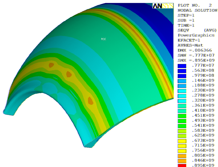
Рис. 13. Эквивалентные напряжения, Па
