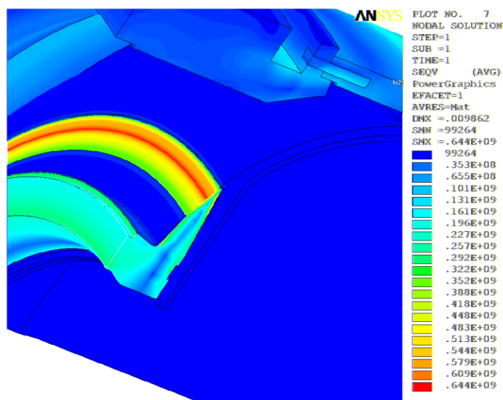
Рис. 10. Эквивалентные напряжения, Па
