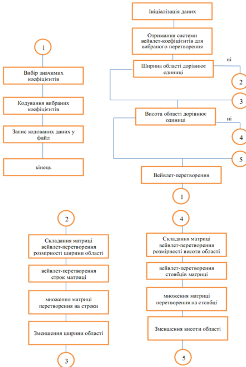
Рис. 1. Алгоритм прямого вейвлет-перетворення
