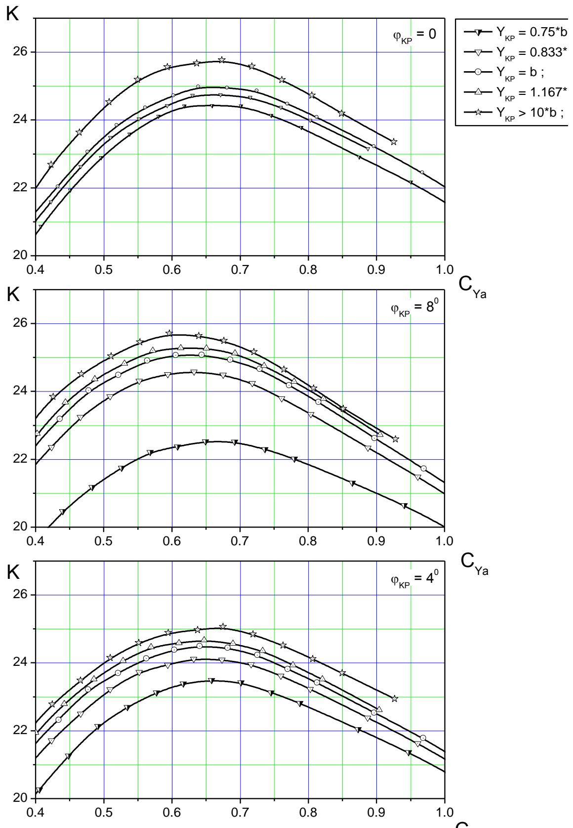
Рис. 4. Зависимости аэродинамического качества K = f(C_{Ya}, \varphi_{кр}, Y_{кр})
