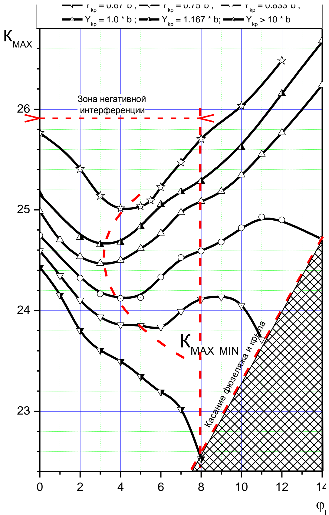
Рис.5. Зависимость K_{max} = f(\phi_{кр}, Y_{кр})
