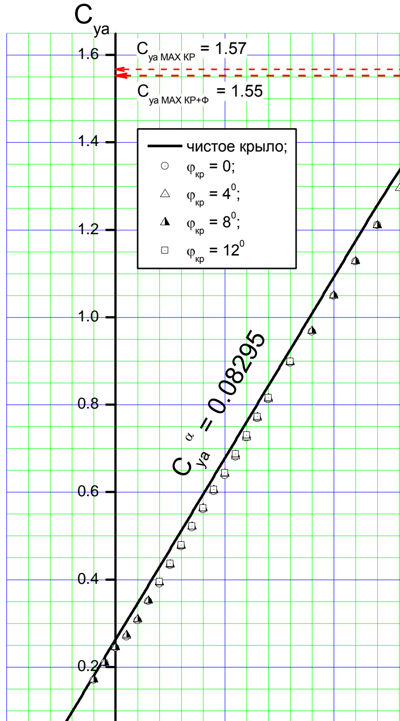
Рис. 3. Зависимости C_{y,a} = f(\alpha, \varphi_{кр}, Y_{кр})
