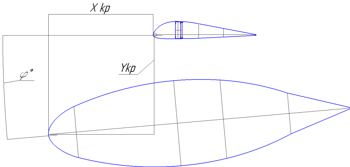
Рис. 1. Параметры \varphi_{кр} , Y_{кр} и X_{кр}
