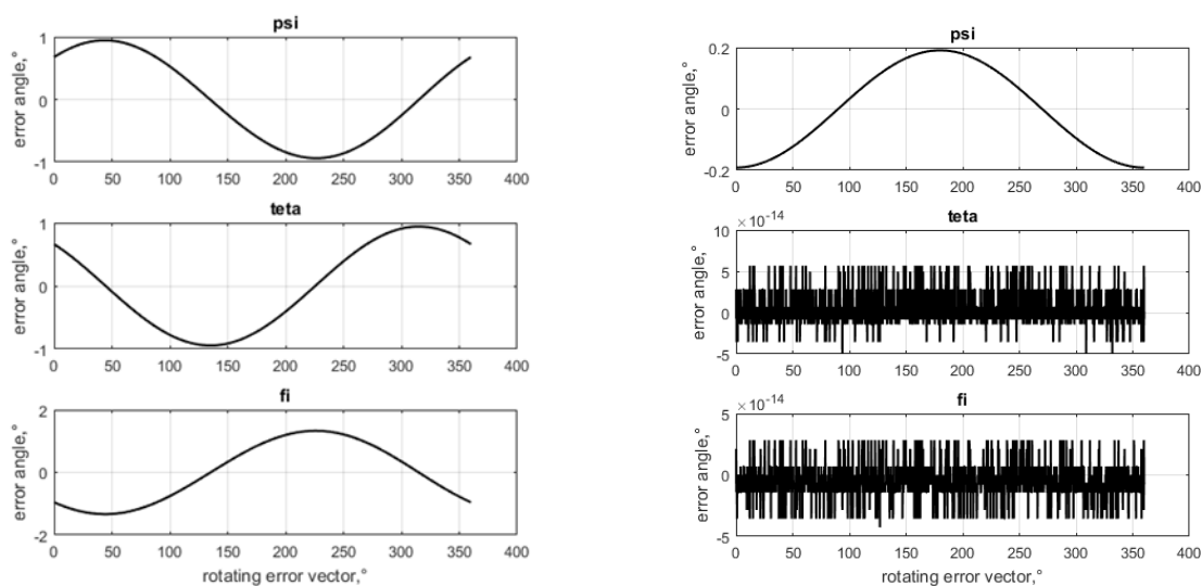
Рис. 6. Влияние неточности НС на нахождение углов ориентации тела при влиянии на опорный и не опорный вектора алгоритма
