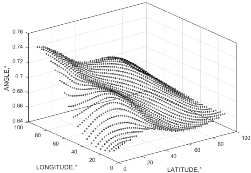
Рис. 5. Распределение погрешности угла на новой выборке
