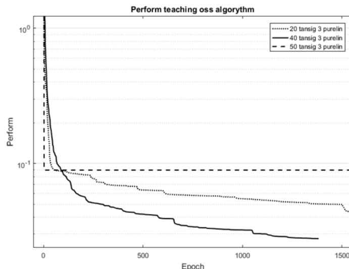
Рис. 4. График скорости обучения алгоритмом «trainoss»
