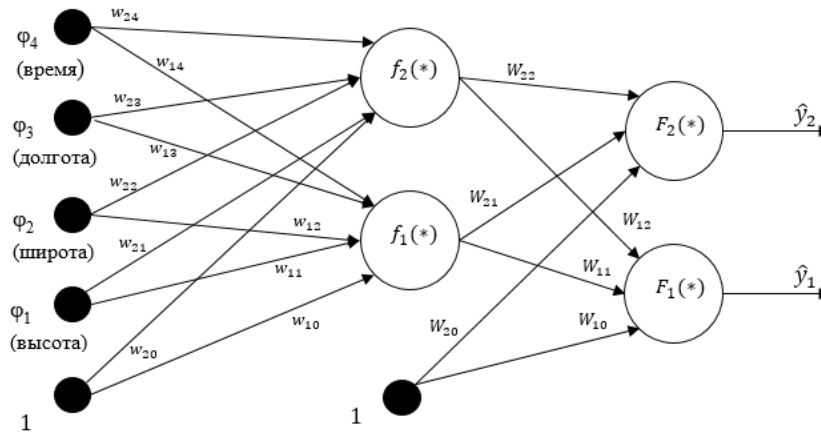
Рис. 1. Схема структуры нейронной сети
