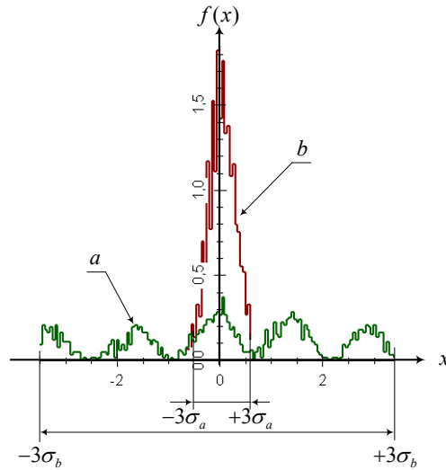
Рисунок 10 - Розподіл щільності імовірності інтегральної нелінійності по діапазону A_{ВНХ}
