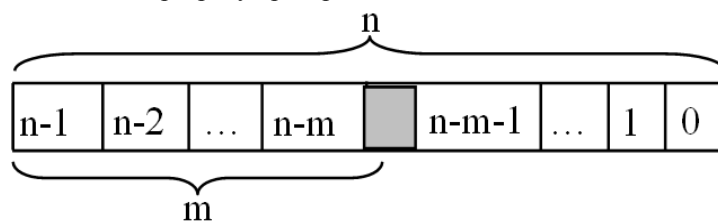
Рисунок 2 - Модель розрядної сітки ЦАП у режимі цифрового самокалібрування
