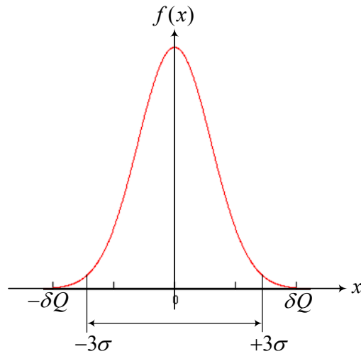
Рисунок 3 - Щільність розподілу технологічного допуску \delta Q
