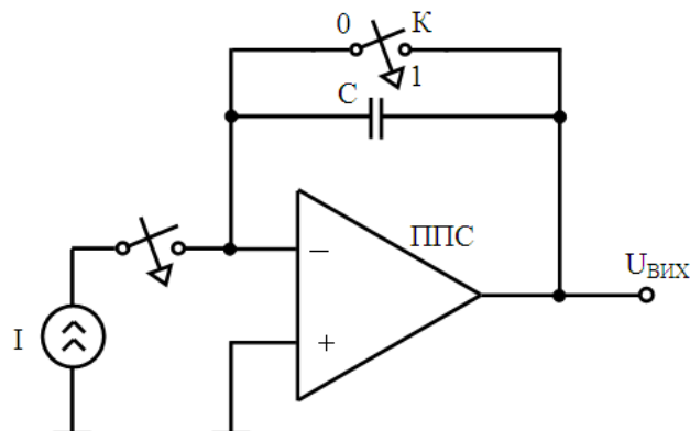
Рисунок 6 - Схема ГКС
