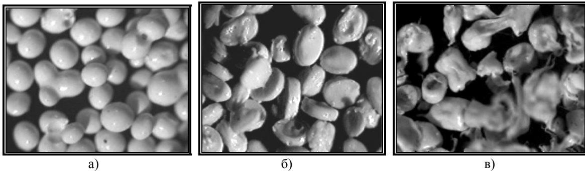
Рисунок 3 – Изменение формы гранул при различных значениях концентрации лака: а) c = 10\% ; б) c = 20\% ; в) c = 28\%
