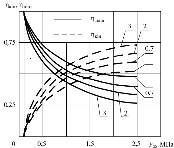
Рисунок 2 – Криві розподілу наявної енергії на зрізі сопла на \eta_{кін} та \eta_{тепл} залежно від \alpha_T та P_k (цифрами на кривих наведено значення \alpha_T )
