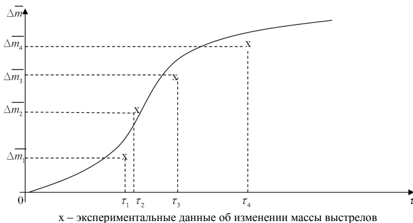
Рисунок 2 – Уменьшение массы порохового заряда при хранении
