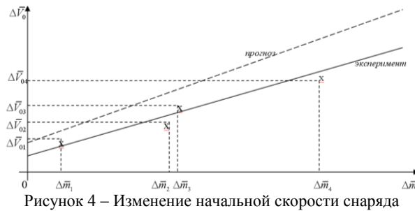
Рисунок 4 – Изменение начальной скорости снаряда
