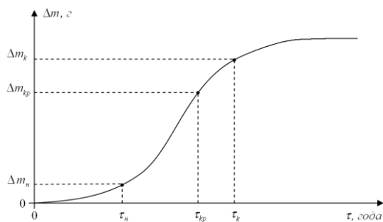
Рисунок 1 – Потеря массы порохового заряда
