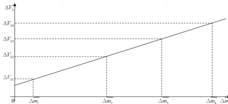
Рисунок 3 – Изменение начальной скорости снаряда в функции от изменения массы выстрела
