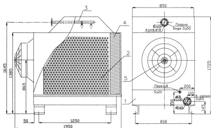
Рисунок 2 – Градирня ГМВ – 10П
