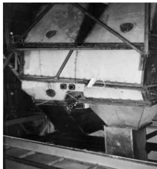
Рисунок 3 – Тепломассоутилизатор ТГ-2-200
