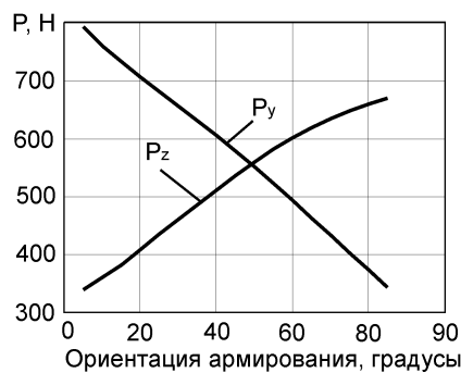
Рисунок 2 – Розраховані значення сил різання
