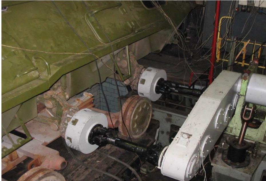
Рисунок 2 – Подключение суммирующего редуктора к ступицам колёс задних мостов бронетранспортера с помощью карданных валов и переходников
