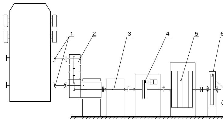
Рисунок 1 – Схема сборки нагружающего устройства для испытаний колёсных БТР (на один борт)
