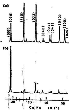
Рисунок 5 – Дифракційні картини рентгеновських лучей для поверхності спечених изделий: а – обычное прессование измельченных порошков; б – прессование многослойных пакетов из пластин, сформированных из порошков с частицами продолговатой формы
