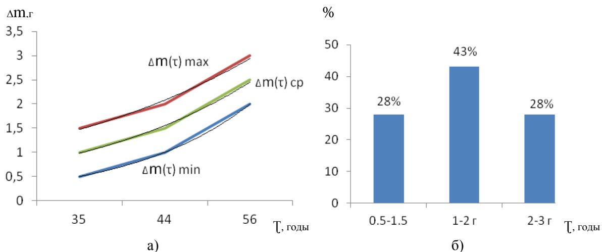
Рисунок 1 – а) изменение массы основного метательного заряда минометной системы 2-С-12 в зависимости от срока хранения. б) доли диапазонов изменения массы основного метательного заряда
