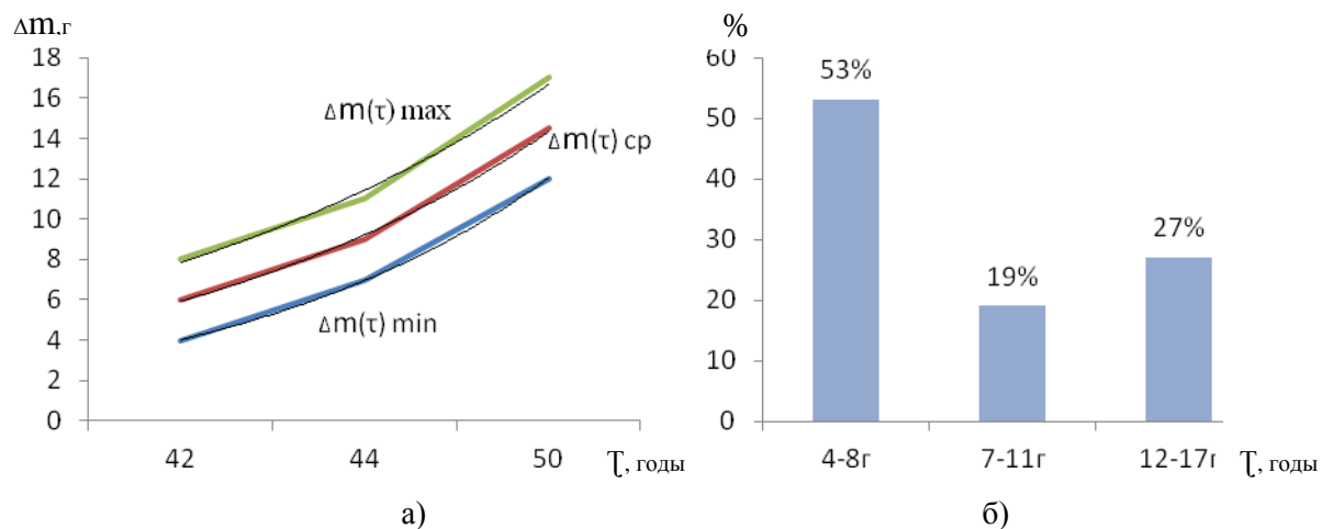
Рисунок 2 – а) изменение массы дополнительного метательного заряда (дополнительных пучков) минометной системы 2-С-12 в зависимости от срока хранения, б) доли диапазонов изменения массы дополнительного метательного заряда
