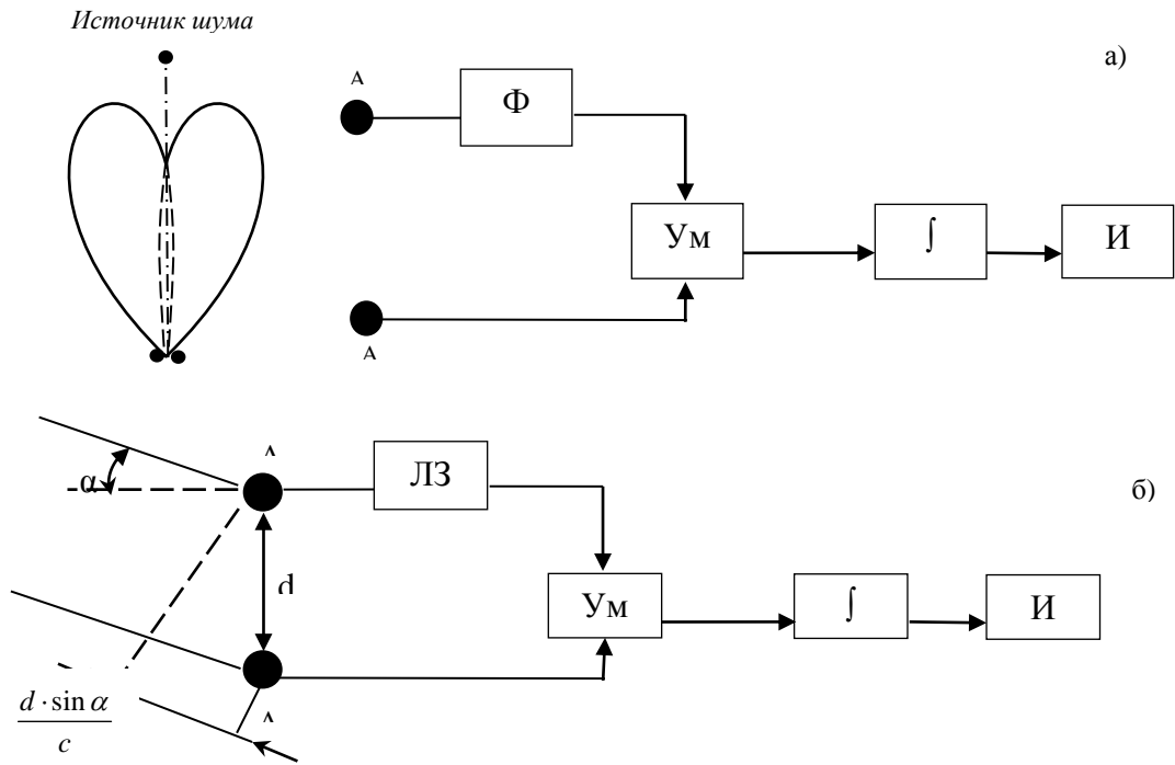
Рисунок 3 – Схемы пеленгаторов:
