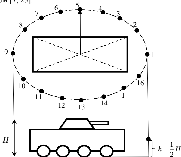
Рисунок 2 – Схема расположения измерительных микрофонов
