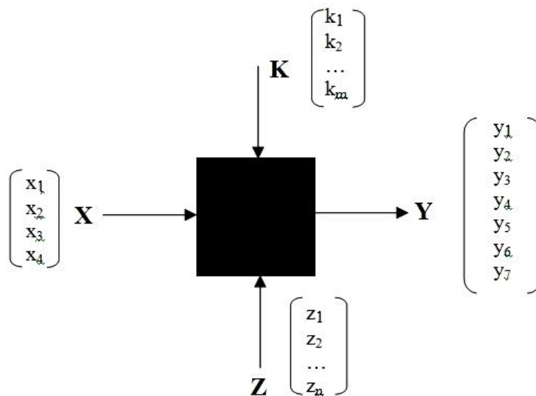
Рис. 4. Математична модель експерименту у вигляді «чорної скриньки»: X — матриця вхідних змінних; Y — матриця функцій відгуку; K , Z — матриці збудуючих [контрольованих, некерованих ( K ) та неконтрольованих, некерованих ( Z )] змінних.
