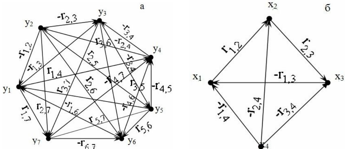
Рис. 5. Граф кореляційних зв'язків між y_i \sim y_j (а) та x_k \sim x_m (б).
