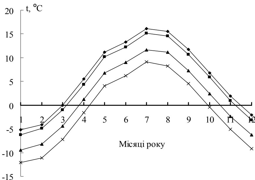
Рис. 1. Середньомісячні температури в локалітетах Pinus cembra , мінімум і максимум поширення температур за місяцями року і за висотою над рівнем моря: 1 – 700 м (південний захід); 2 – 700 м (північний схід); 3 – 1700 м (південний захід); 4 – 1570 м (північний схід).
