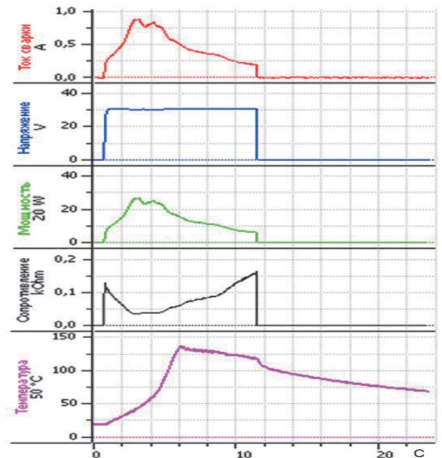
Рис. 7. Осцилограми параметрів режиму зварювання леголі. Електрокоагулятор ЕК300М1
