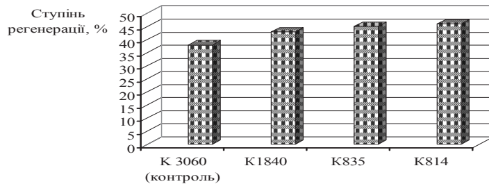
Рис. 2. Залежність ступеню регенерації АВ від марки АВ Silcarbon
