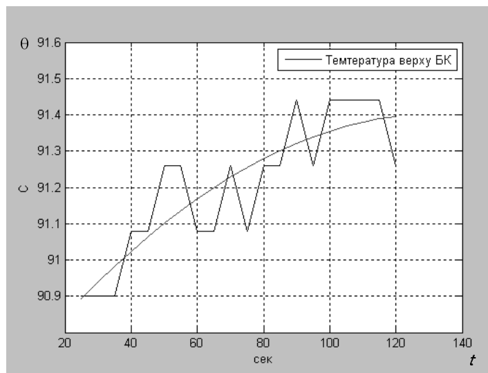
Рис. 2. Тренд температури верху бражної колони (БК)
