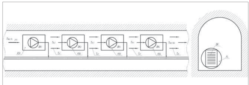
Рис. 1. Схема руху теплових потоків від модулів ПМКС і вентиляційного повітря в гірничій виробці (КУі – компресорні установки (модулі) в складі ПМКС; ВКі – гвинтові компресори в складі модулів; Ті – температури потоків)
