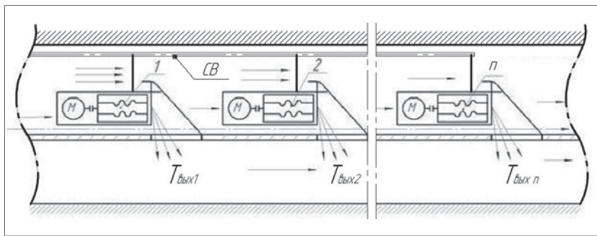
Рис. 3. Технологічна схема ПМКС з відводом теплових потоків від модулів
