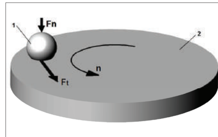
Рис. 1. Схема пары трения трибологического тестера Т-01 М: 1 – шарик, 2 – диск
