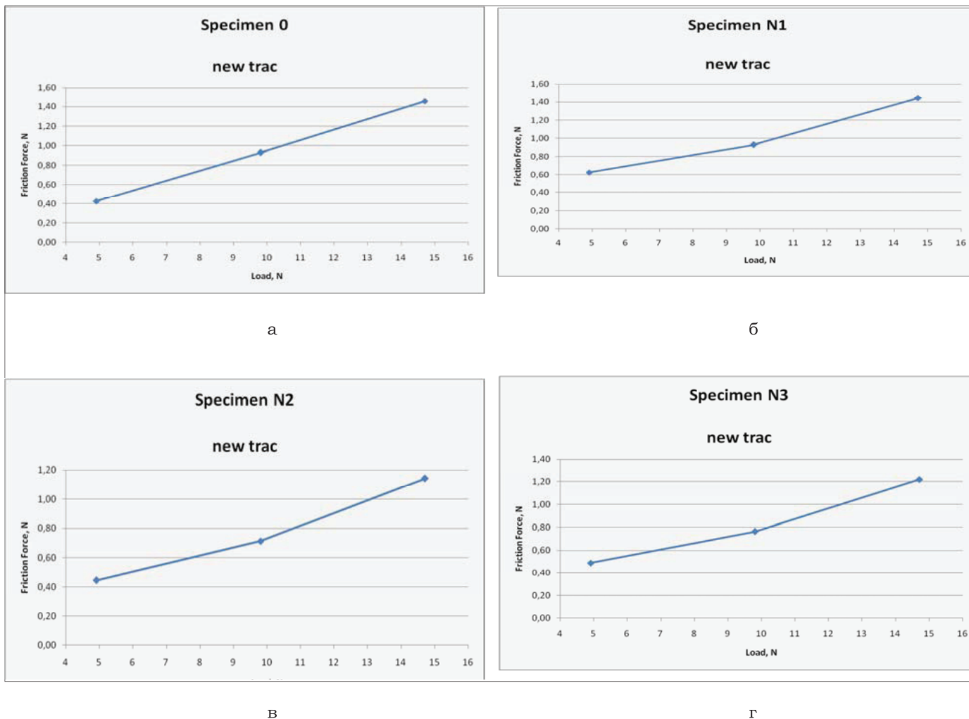
Рис.10. Изменение силы трения стального шарика по поверхности бронзового диска при различных нагрузках: а – серия 0; б – серия № 1; в серия № 2; г – серия № 3
