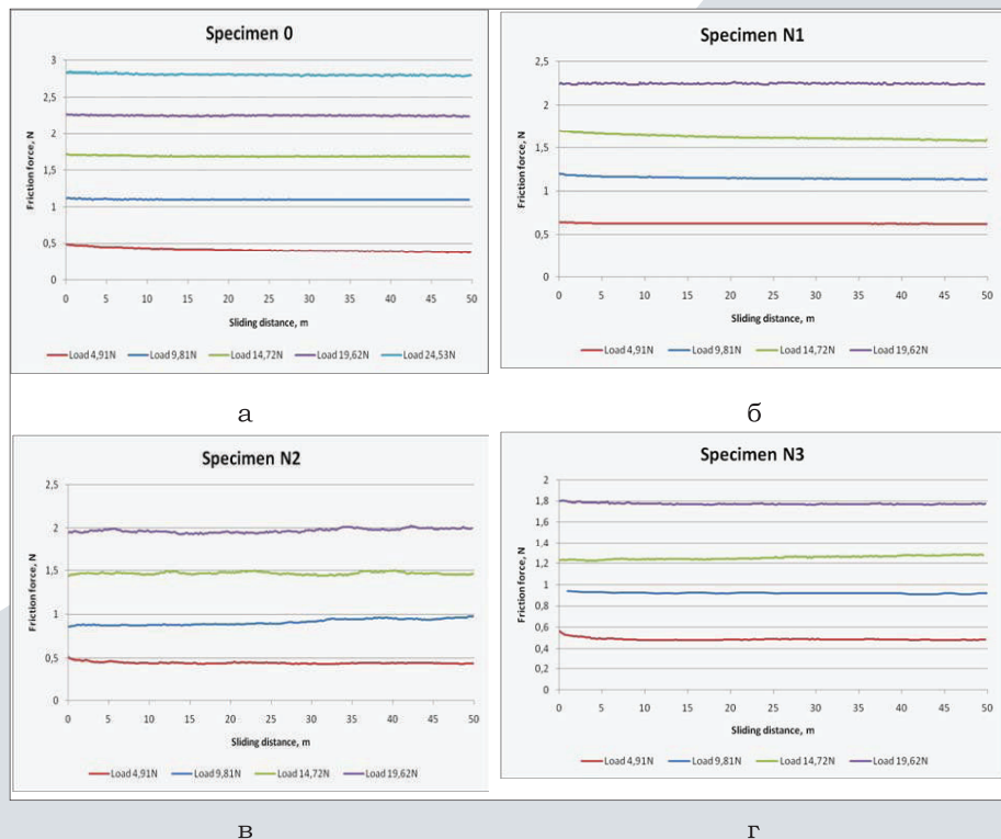
Рис. 8. Изменение силы трения стального шарика по поверхности бронзового диска при различных нагрузках: а – серия 0; б – серия № 1; в серия № 2; г – серия № 3
