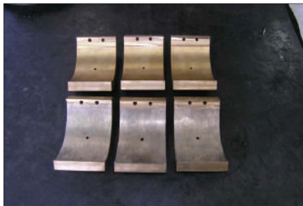
Рис. 3. Бронзовые вкладыши подшипников скольжения
