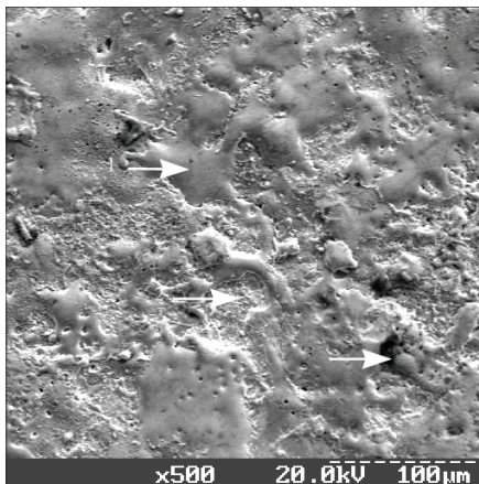
Рис. 4. Топография участка поверхности образца с КЭП из серебра, меди и баббита Б83
