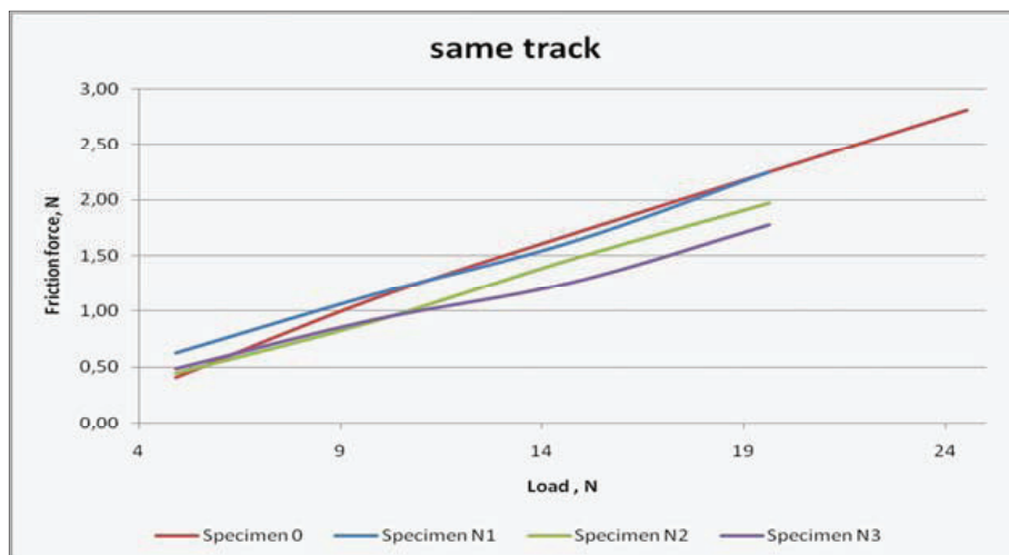
Рис. 9. Зависимость силы трения от нагрузки
