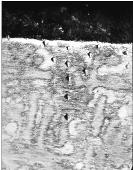
Рис. 7. Микроструктура и распределение микротвердости поверхностного слоя образца из бронзы ОЦС 5-5-5
