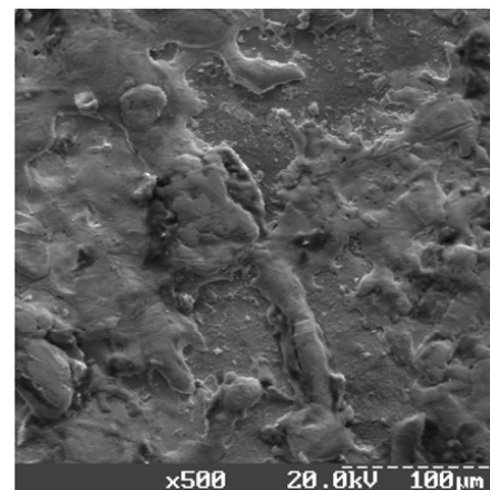
Рис. 5. Изображение поверхности бронзового образца с КЭП во вторичных электронах
