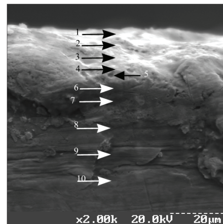
Рис. 6. Точки сканирования поэлементного состава покрытия по глубине слоя
