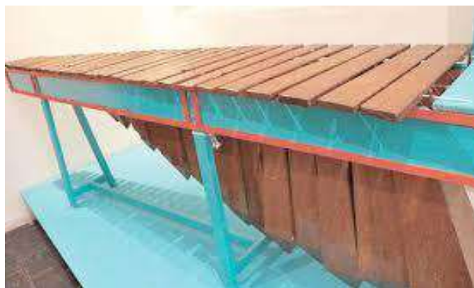
Рис. 2. Маримба "sencilla"
